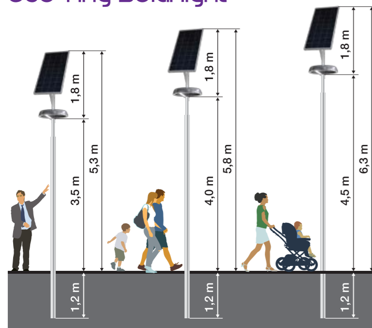
Wymiary zestawów Eco-Ring SolarLight
